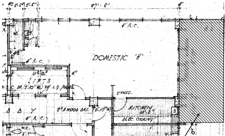
7/F Plan 7字樓平面圖
