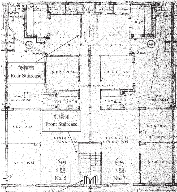
G/F Plan 地下平面圖
