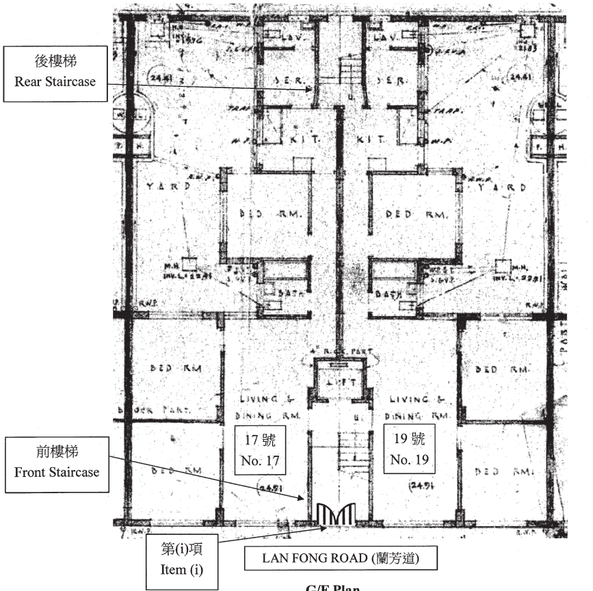
G/F Plan 地下平面圖
