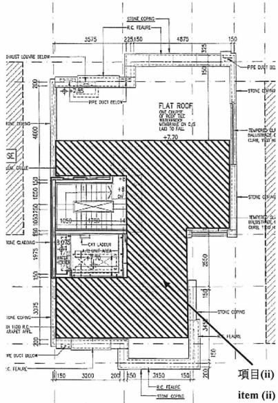
R/F Plan (天台平面圖) item (ii)
